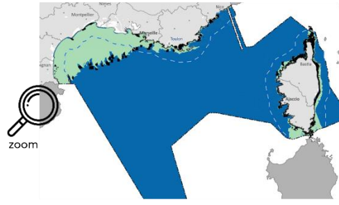
Figure 3. Schéma synthétisant la méthode de spatialisation pour les habitats benthiques
