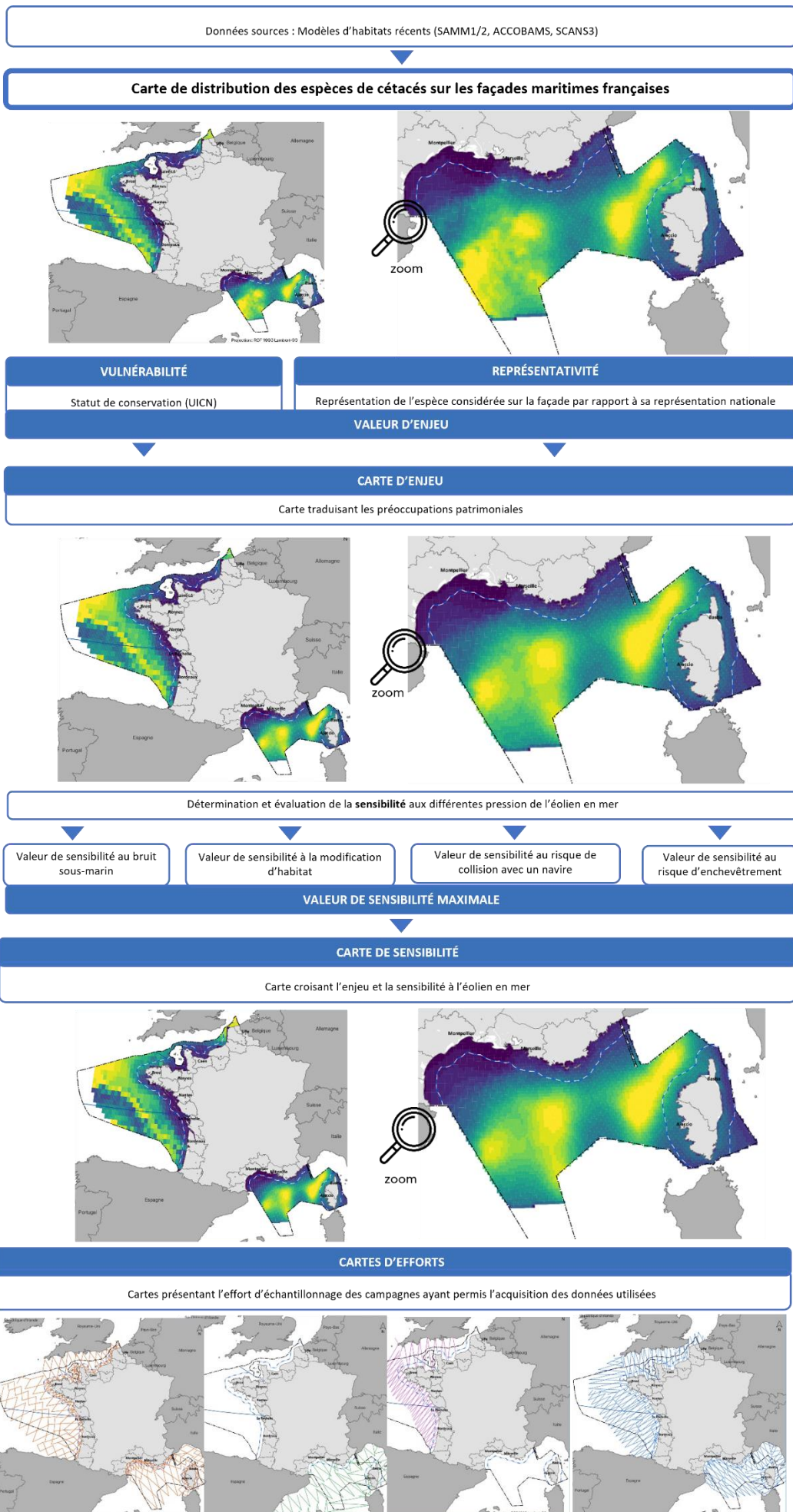
Figure 16. Schéma synthétisant la méthode de spatialisation pour les cétacés
