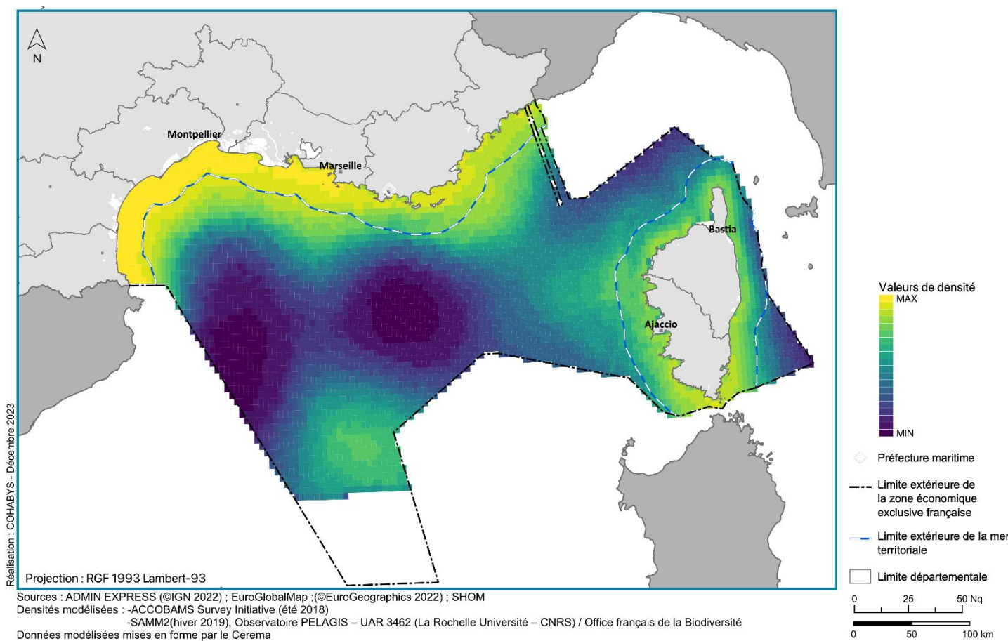
Figure 30. Carte de distribution du fou de Bassan sur la façade
