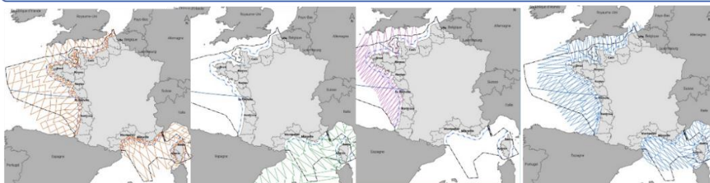
Figure 11. Schéma synthétisant la méthode de spatialisation pour l'avifaune
