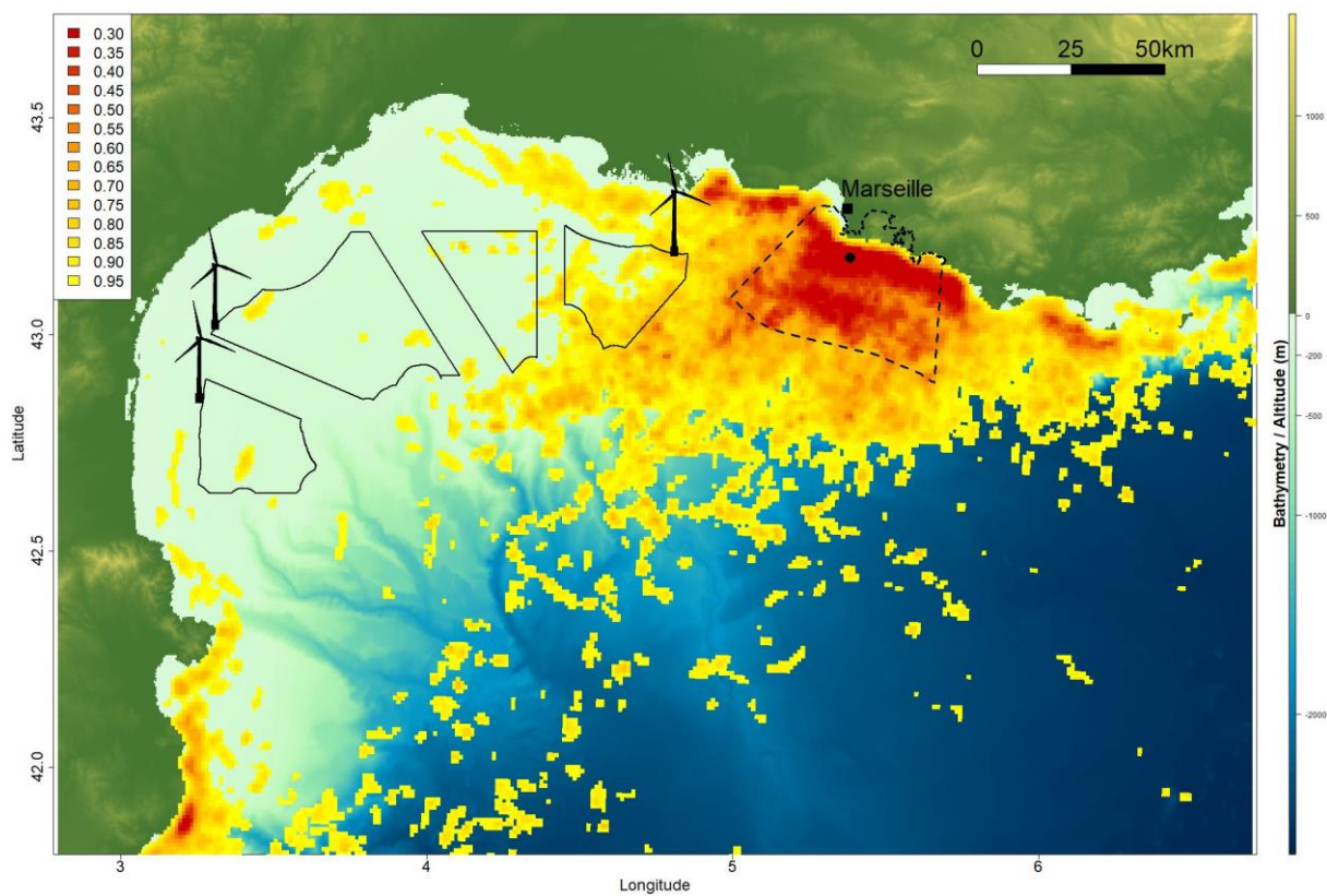
Figure 6 : Caractérisation de l'espace utilisé par les puffins de Scopoli dans le golfe du Lion (à partir des individus équipés dans le cadre du programme Migralion). Les limites du parc national des Calanques sont en pointillé. Les emplacements des trois projets pilotes d'éolien flottant sont indiqués par une éolienne et les quatre zones d'étude pour des projets commerciaux d'éolien flottant par des polygones en traits pleins.
