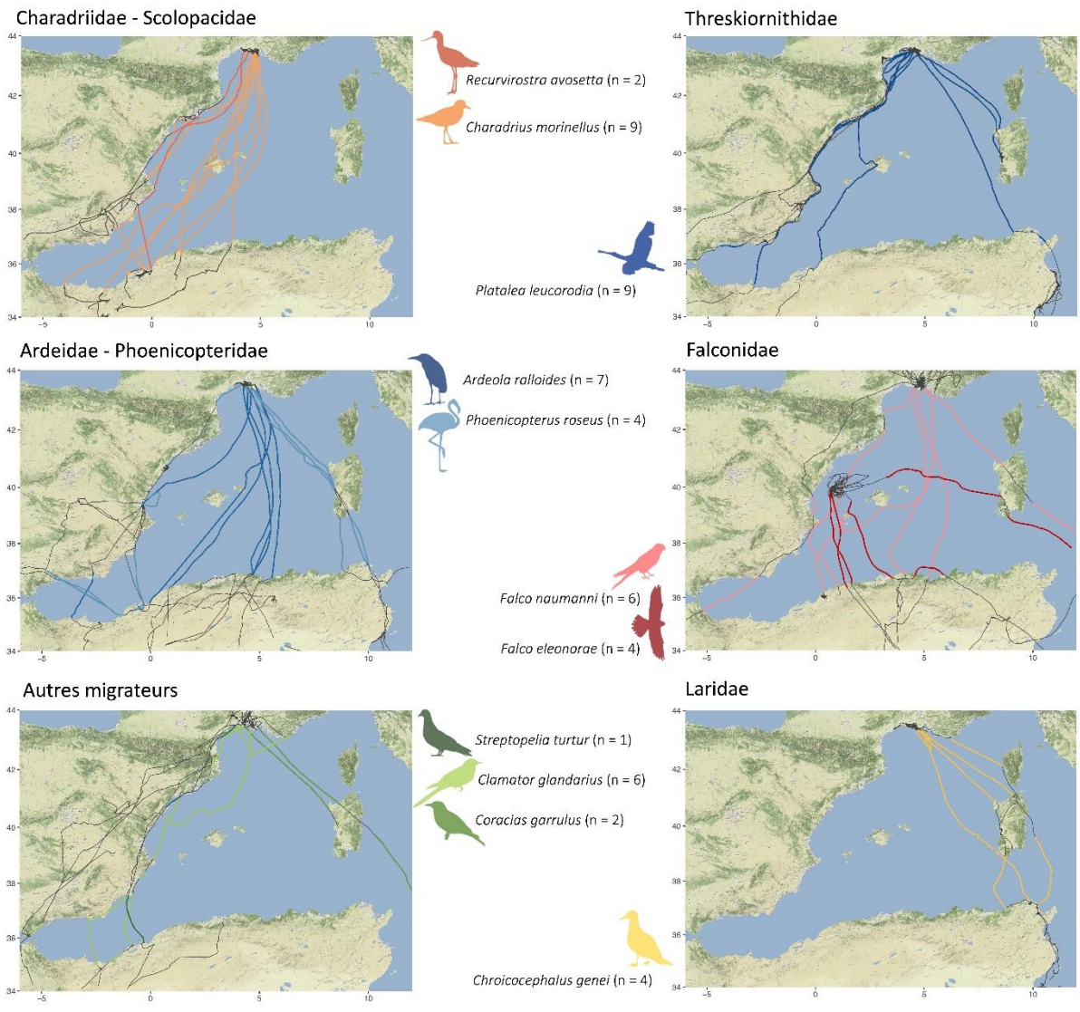
Figure 5 : Déplacements des oiseaux terrestres équipés de balises GPS dans le cadre du programme Migralion qui ont entrepris des migrations en mer (leur nombre par espèce est indiqué entre parenthèses). Les espèces sont regroupées par famille.
