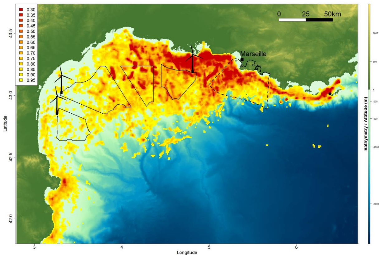
Figure 8 : Caractérisation de l'espace utilisé par les puffins yelkouan dans le golfe du Lion (à partir des individus équipés dans le cadre du programme Migralion). Les limites du parc national des Calanques sont indiquées en pointillé. Les emplacements des trois projets pilotes d'éolien flottant sont indiqués par une éolienne et les quatre zones d'étude pour des projets commerciaux d'éolien flottant par des polygones en traits pleins.
