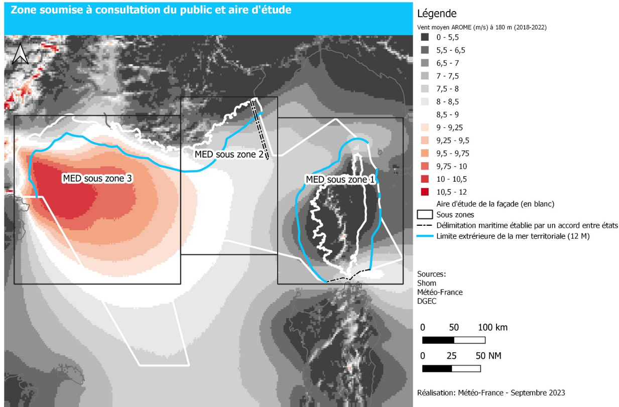
Illustration 25: Carte des vents moyens AROME à 180 m sur la façade MED
