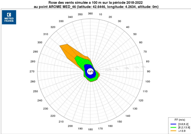
Illustration 24: Rose des vents à 100 m au point MED_46
