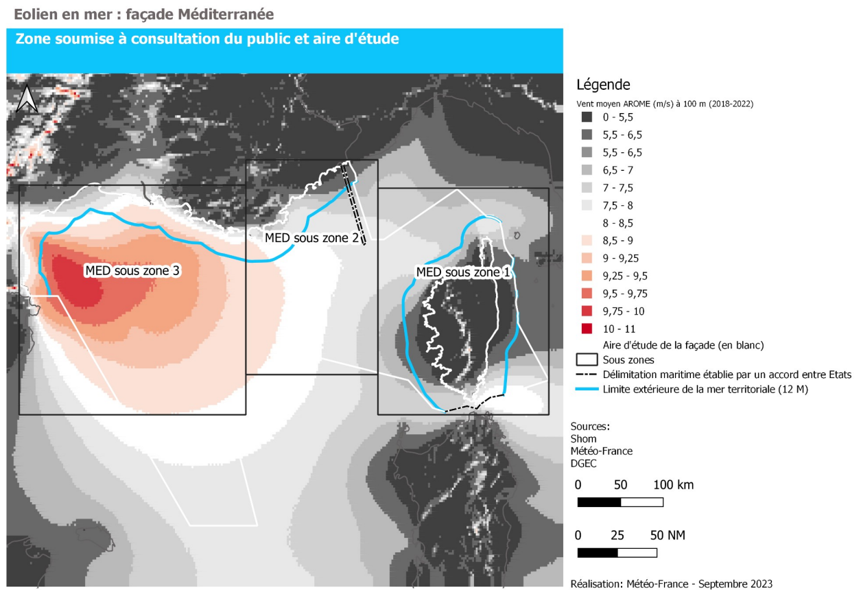
Illustration 15: Carte du vent moyen AROME (m/s) à 100 m sur la façade MED
