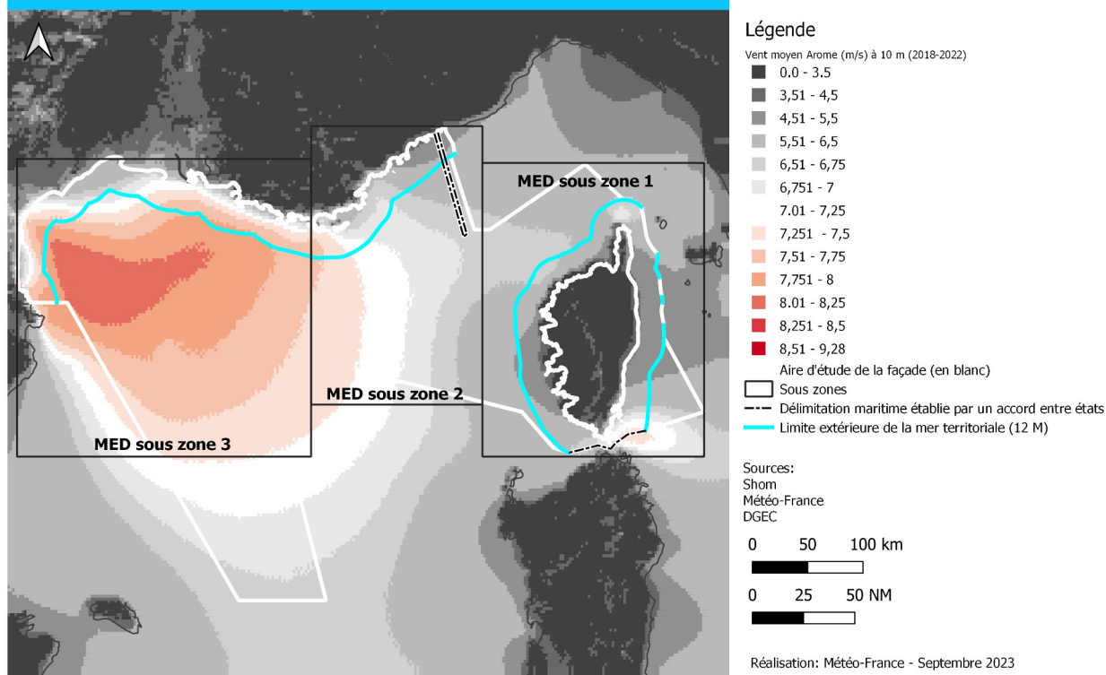
Illustration 5: Carte du vent moyen AROME à 10 m sur la façade MED
