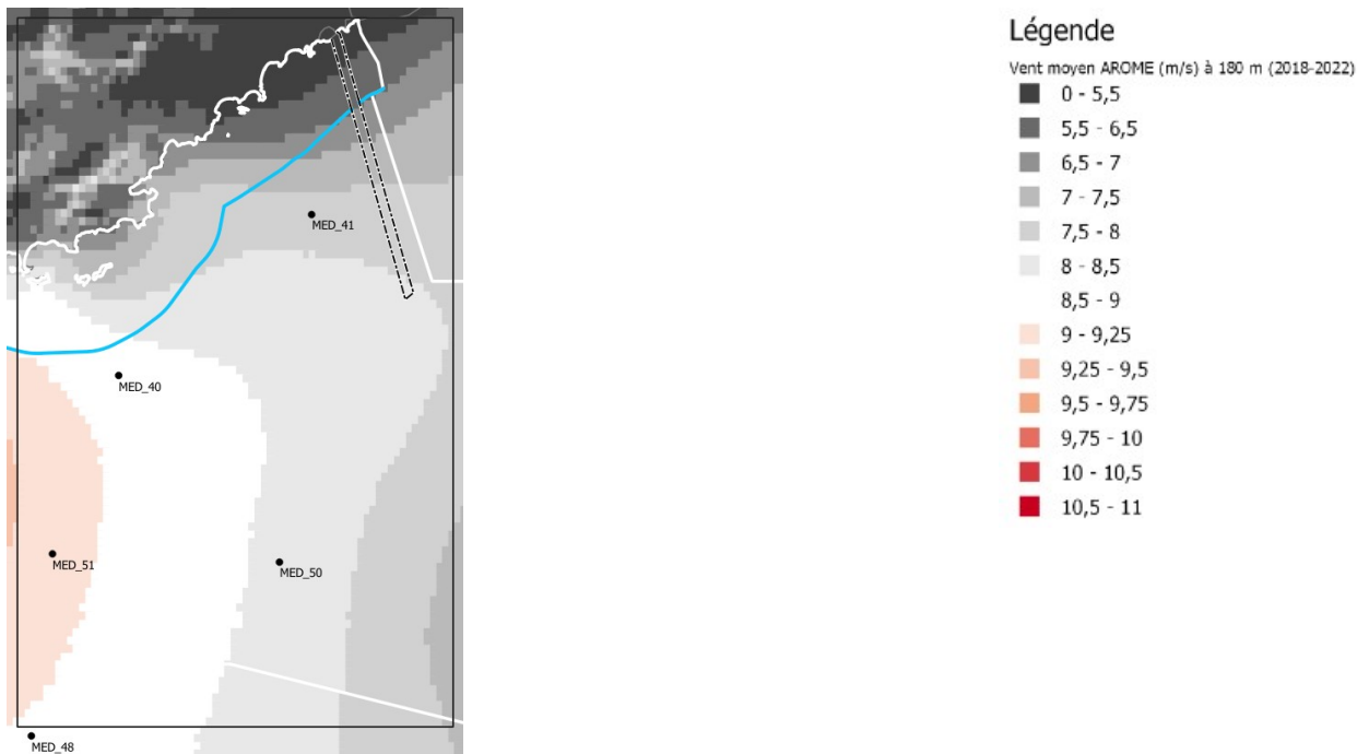
Illustration 27: Champ de vent moyen à 180 m : focus sur la sous-zone 2 de la façade MED
