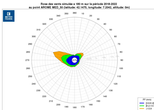
Illustration 33: Rose des vents à 180 m au point MED_50
