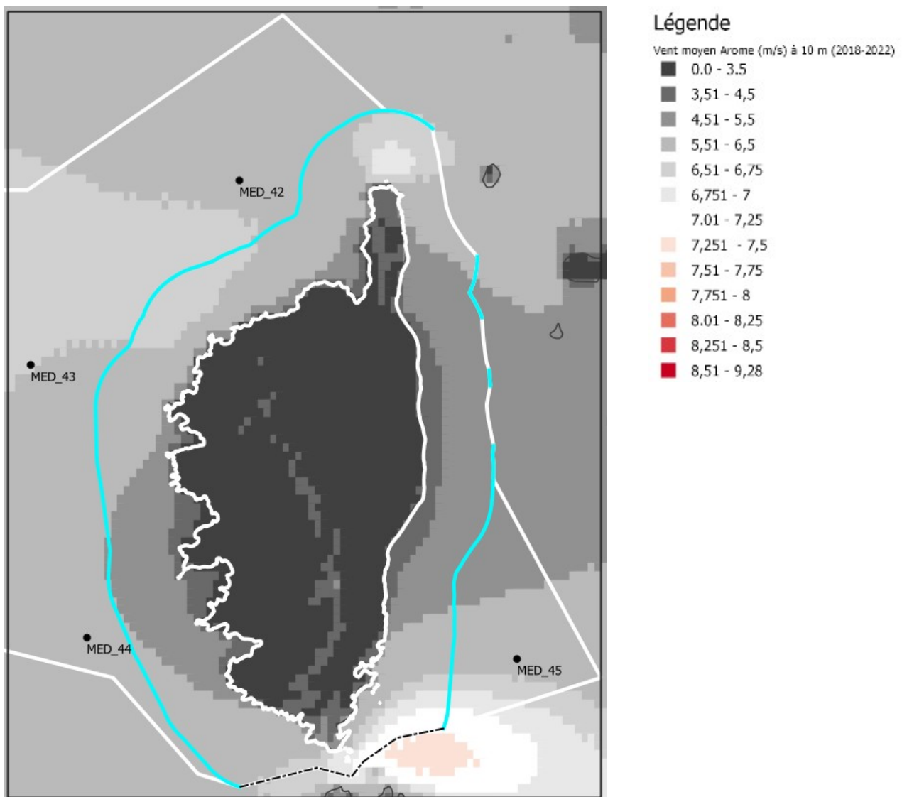
Illustration 6: Champ de vent moyen à 10 m : focus sur la sous-zone 1 de la façade MED
