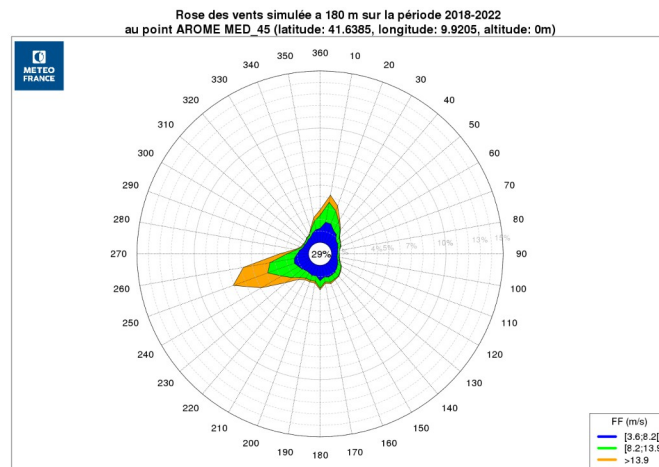
Illustration 32: Rose des vents à 180 m au point MED_45
