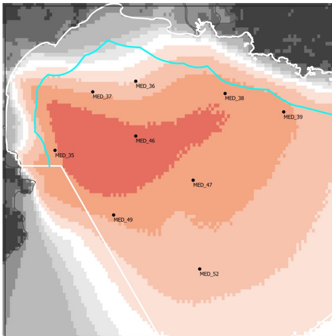
Illustration 8: Champ du vent moyen à 10 m : focus sur la sous-zone 3 de la façade MED
