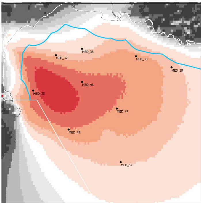
Illustration 18: Champ de vent moyen à 100 m : focus sur la sous-zone 3 de la façade MED
