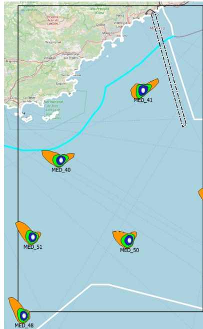
Illustration 10: Roses des vents à 10 m : focus sur la sous-zone 2 de la façade MED
