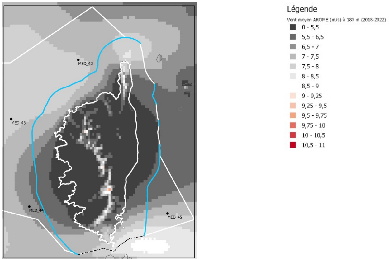
Illustration 26: Champ de vent moyen à 180 m : focus sur la sous-zone 1 de la façade MED
