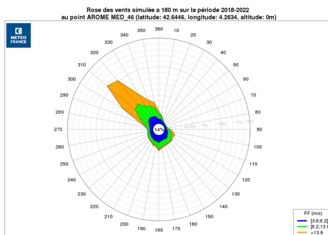
Illustration 34: Rose des vents à 180 m au point MED_46
