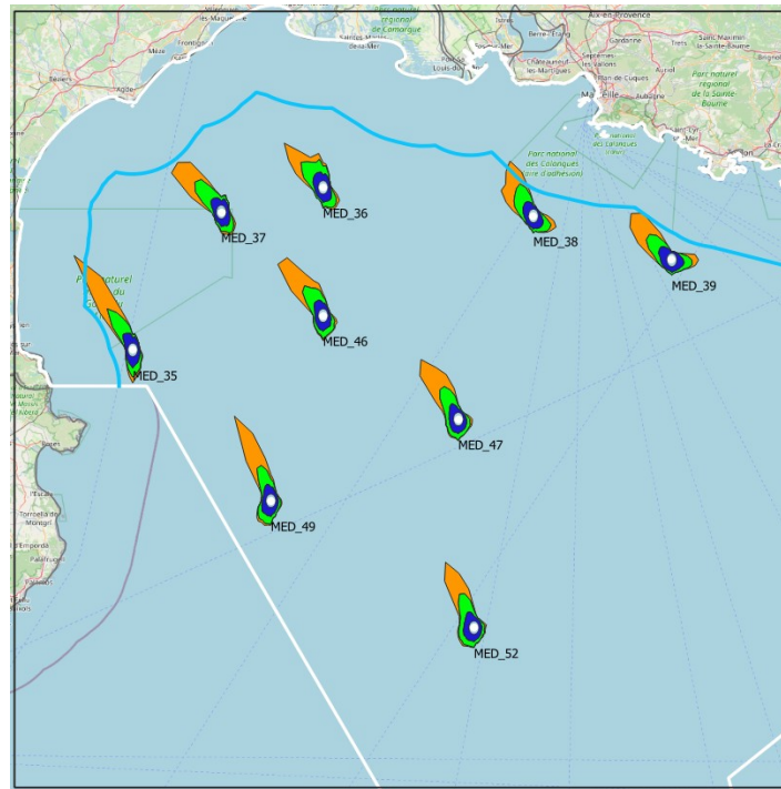
Illustration 31: Roses des vents à 180 m : focus sur la sous-zone 3 de la façade MED
