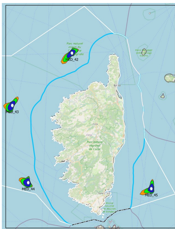
Illustration 19: Roses des vents à 100 m : focus sur la sous-zone 1 de la façade MED
