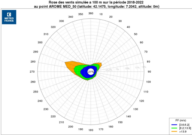
Illustration 23: Rose des vents à 100 m au point MED_50
