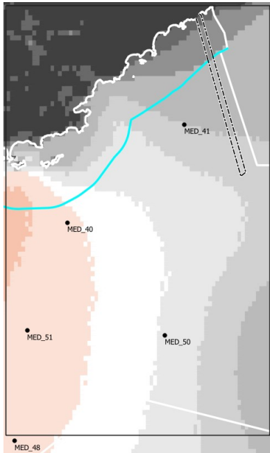
Illustration 7: Champ du vent moyen à 10 m : focus sur la sous-zone 2 de la façade MED
