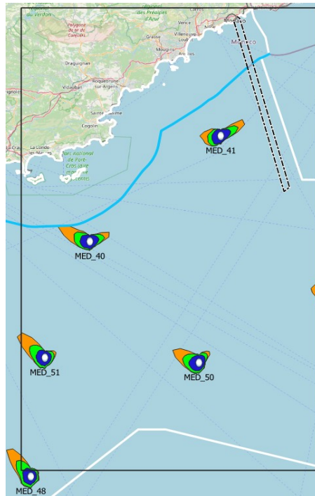
Illustration 30: Roses des vents à 180 m : focus sur la sous-zone 2 de la façade MED
