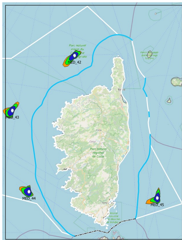
Illustration 29: Roses des vents à 180 m : focus sur la sous-zone 1 de la façade MED
