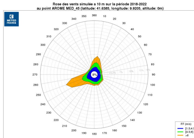
Illustration 12: Rose des vents à 10 m au point MED_45
