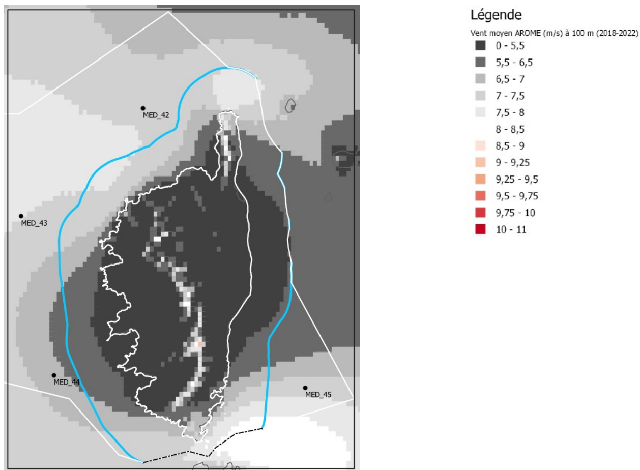
Illustration 16: Champ de vent moyen à 100 m : focus sur la sous-zone 1 de la façade MED
