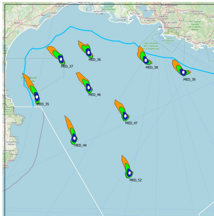
Illustration 21: Roses des vents à 100 m : focus sur la sous-zone 3 de la façade MED
