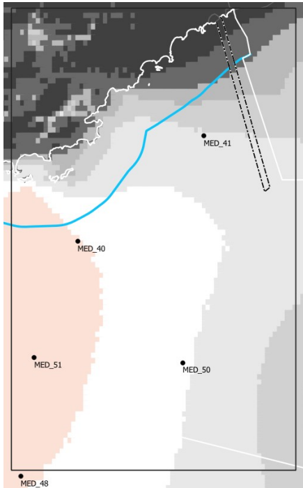
Illustration 17: Champ de vent moyen à 100 m : focus sur la sous-zone 2 de la façade MED
