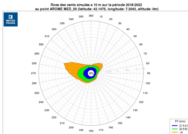
Illustration 13: Rose des vents à 10 m au point MED_50
