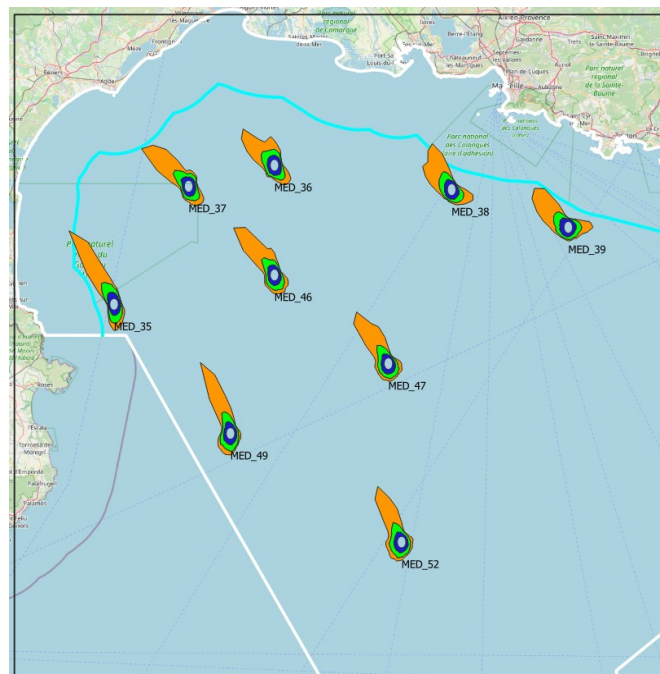
Illustration 11: Roses des vents à 10 m : focus sur la sous-zone 3 de la façade MED
