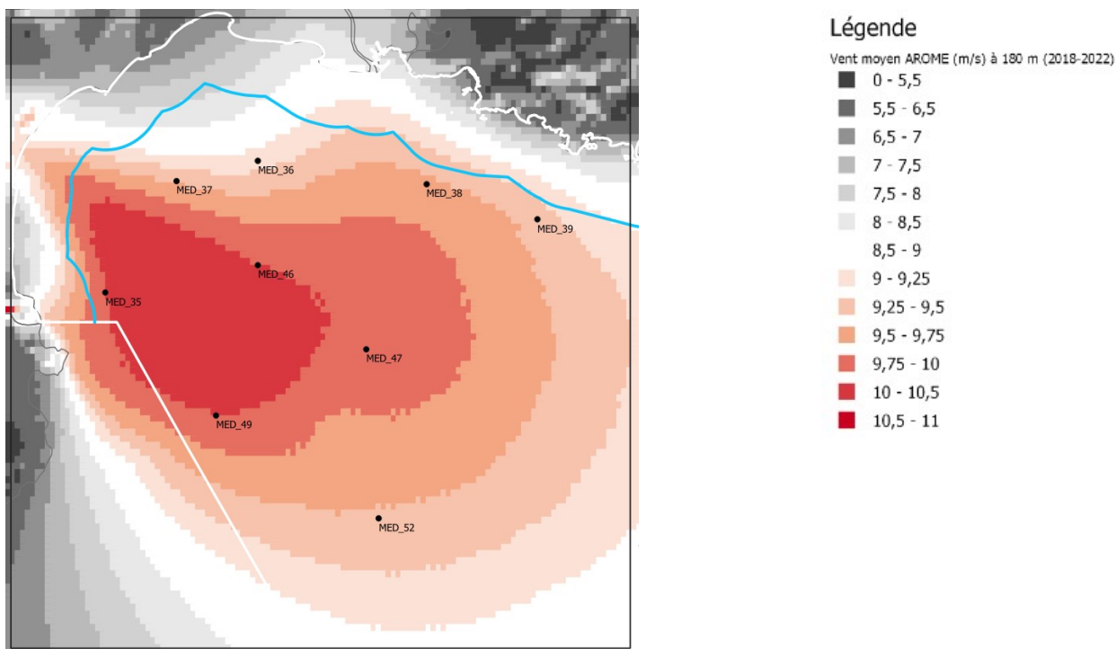
Illustration 28: Champ de vent moyen à 180 m : focus sur la sous-zone 3 de la façade MED
