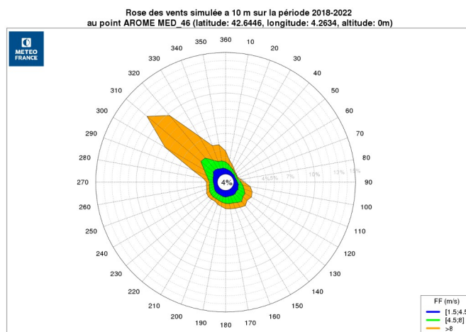
Illustration 14: Rose des vents à 10 m au point MED_46
