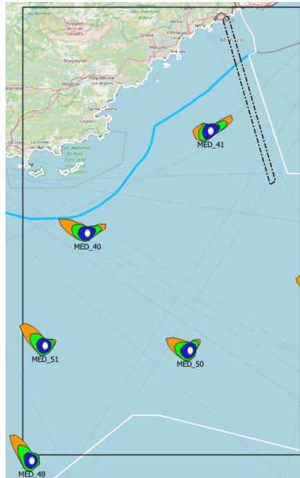
Illustration 20: Roses des vents à 100 m : focus sur la sous-zone 2 de la façade MED
