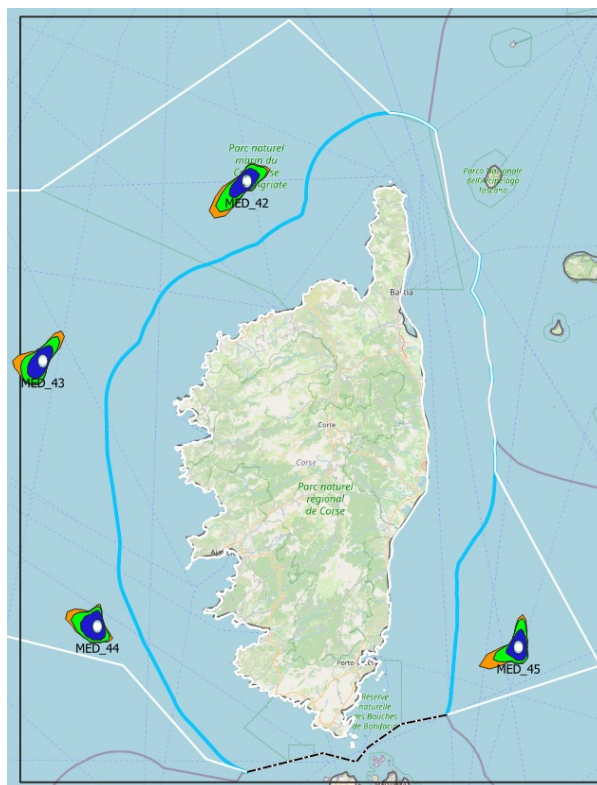
Illustration 9: Roses des vents à 10 m : focus sur la sous-zone 1 de la façade MED
