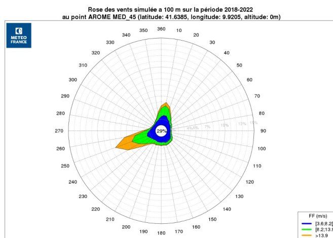
Illustration 22: Rose des vents à 100 m au point MED_45
